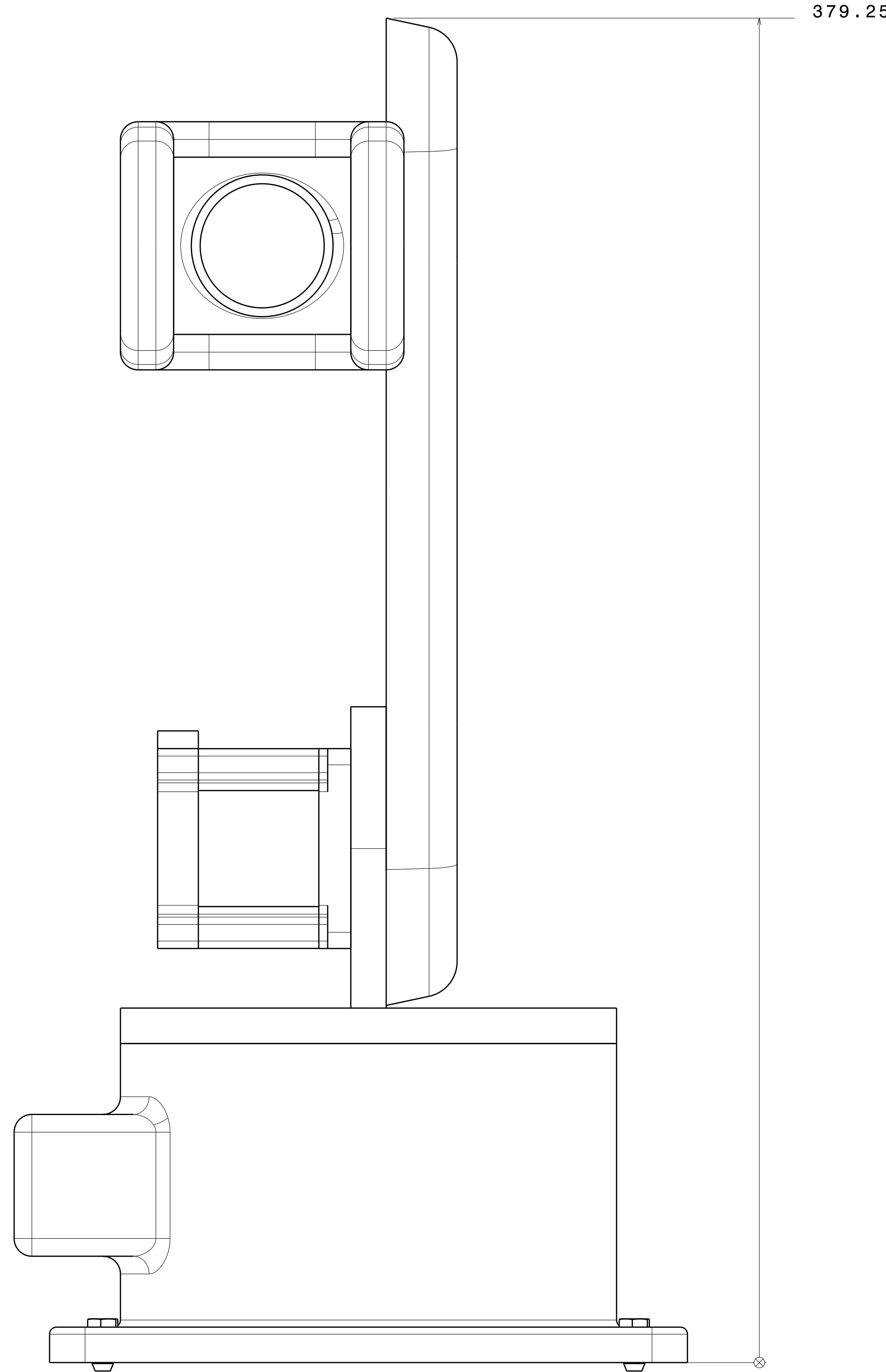
Right view Scale: 1:1
