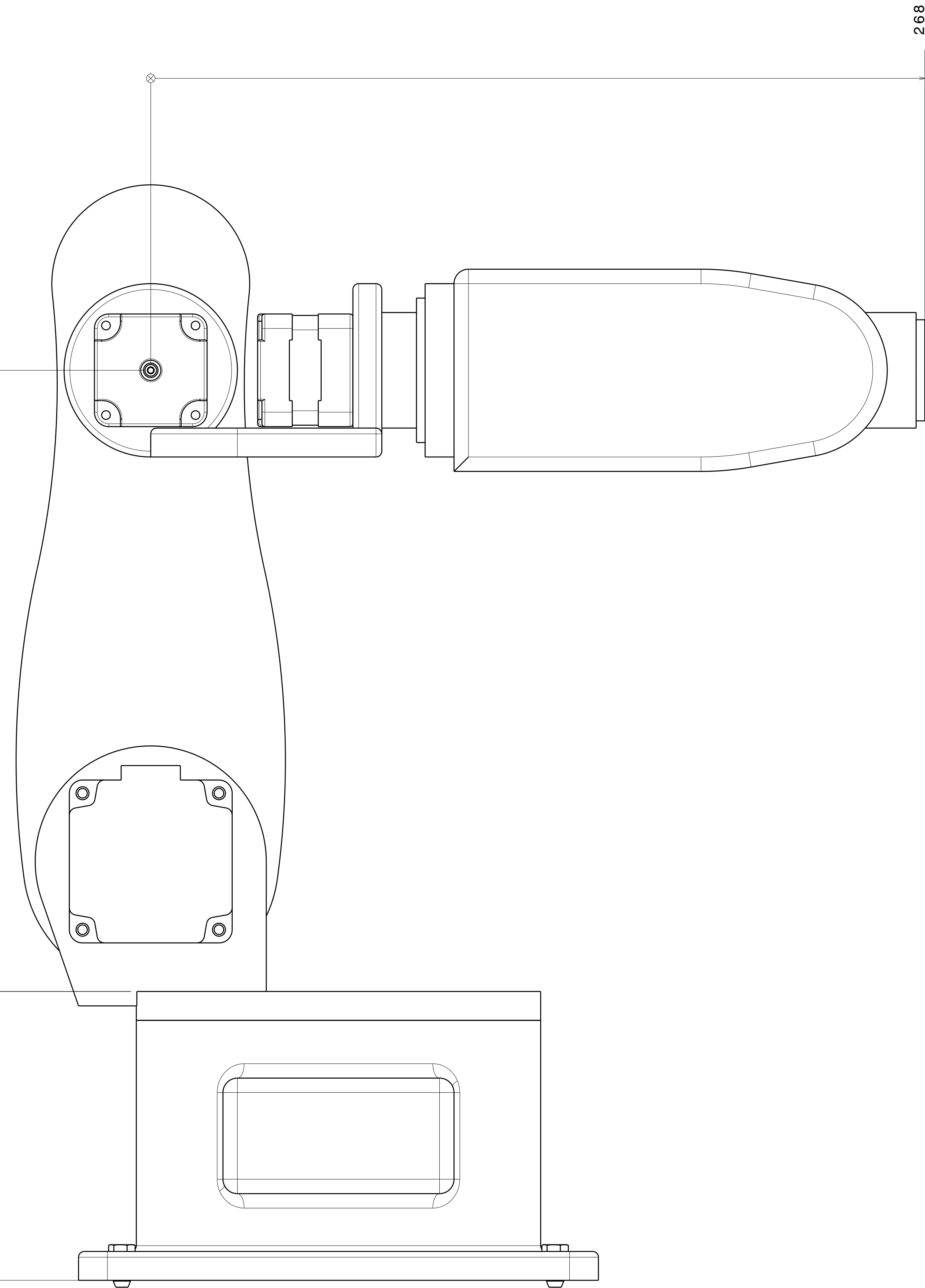
Front view Scale: 1:1
